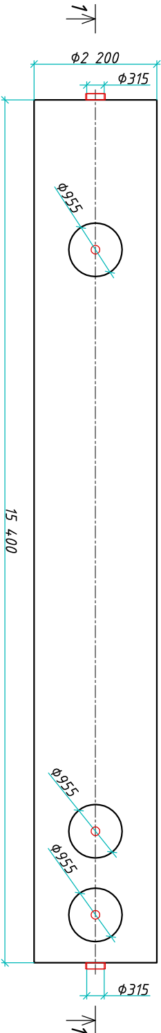
Вид сверху
