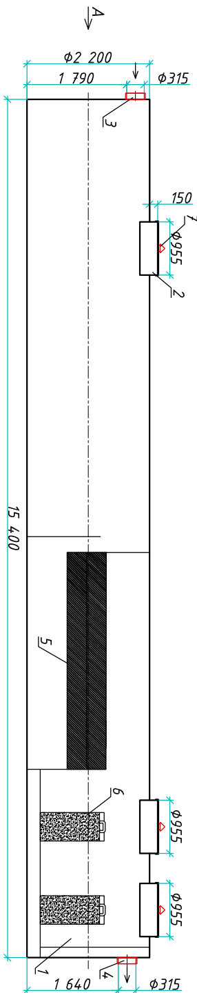
Разрез 1-1
